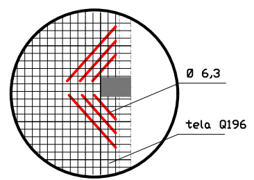
DETALHE ARMADURA COMPLEMENTAR
