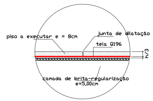
DETALHE PISO
