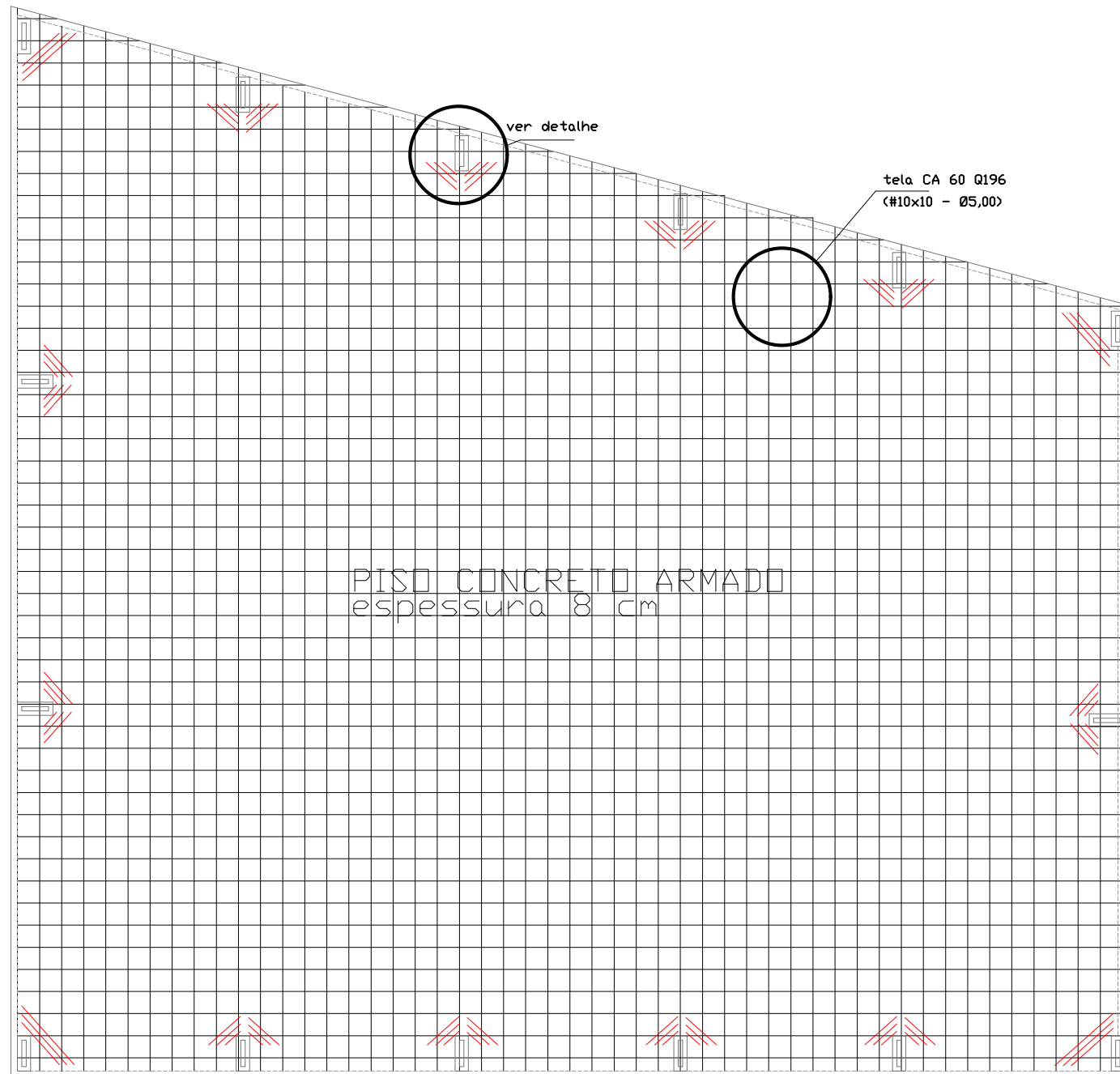
PLANO DE PISO CONCRETO ARMADO
